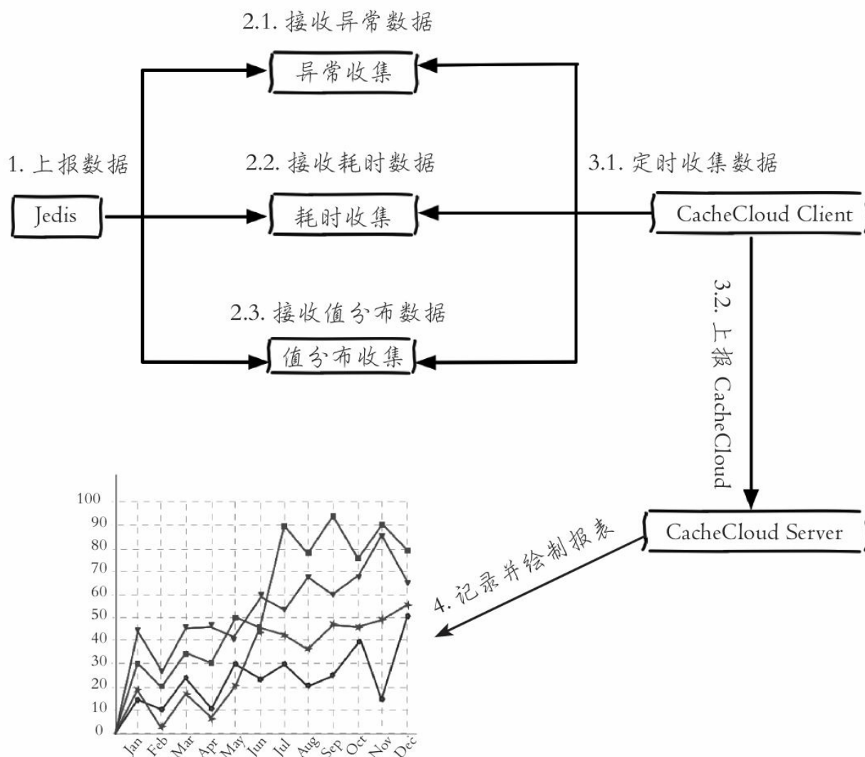
图13-47 客户端上报整体流程
