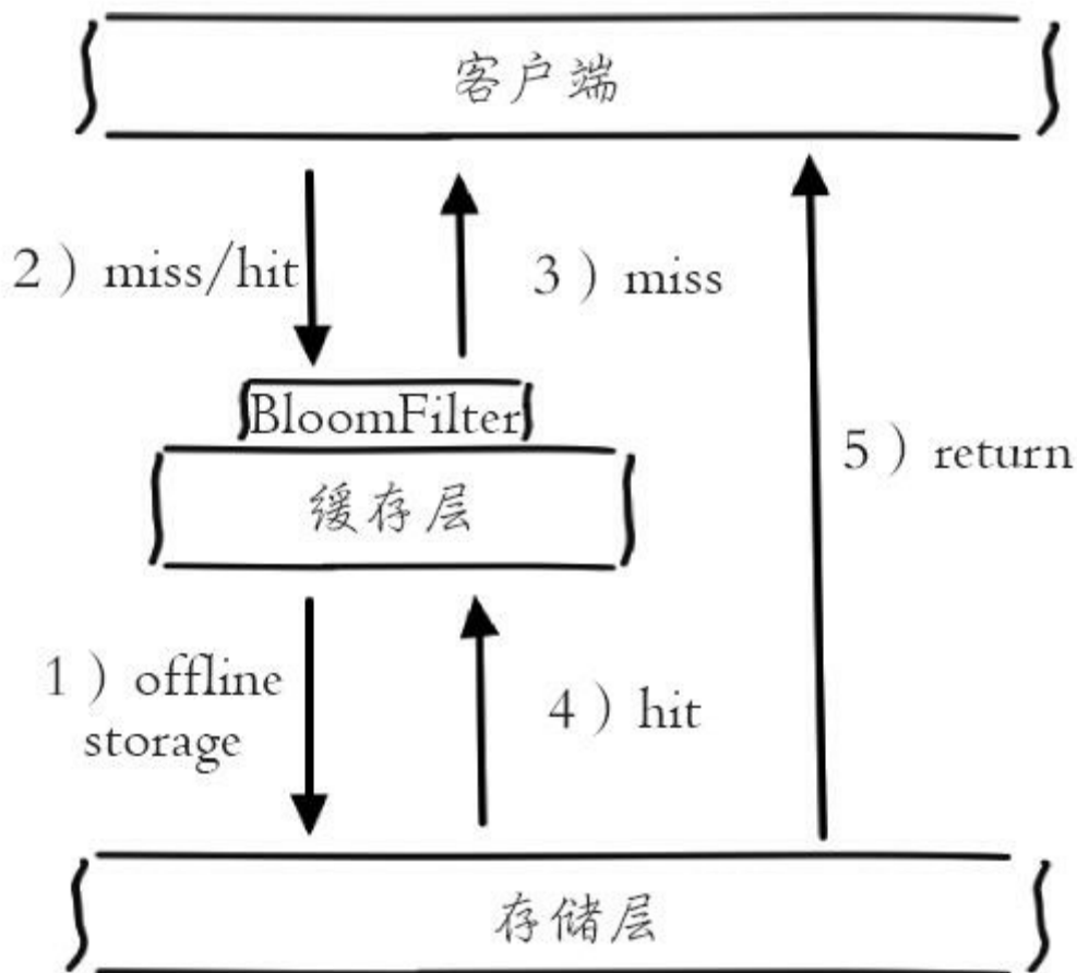
图11-5 使用布隆过滤器应对穿透问题
