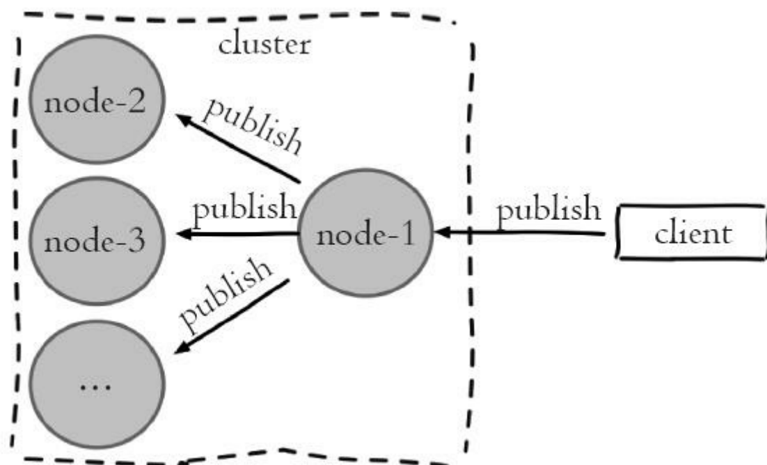
图10-44 publish命令在集群内广播
