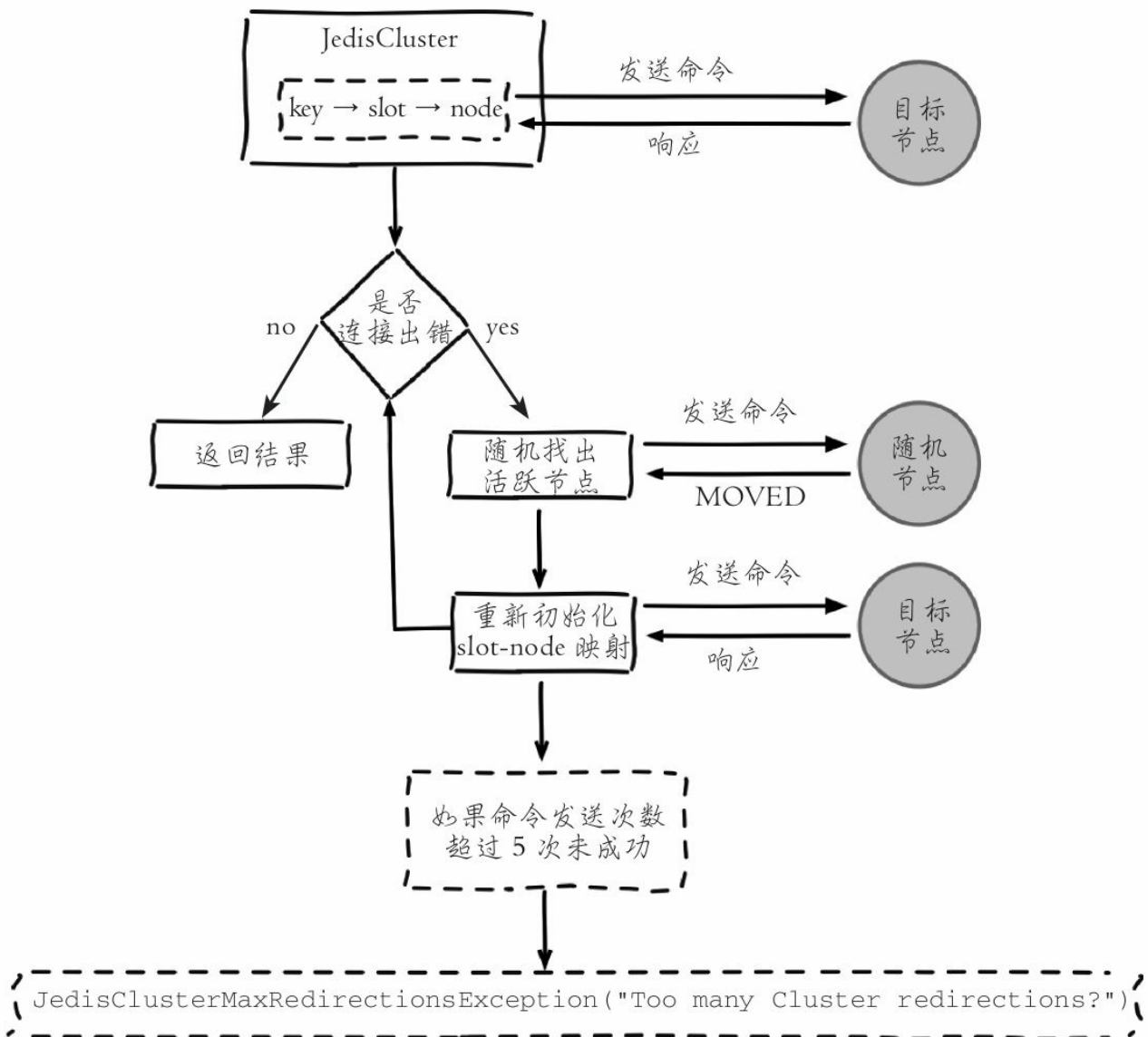
图10-31 Jedis客户端命令执行流程
