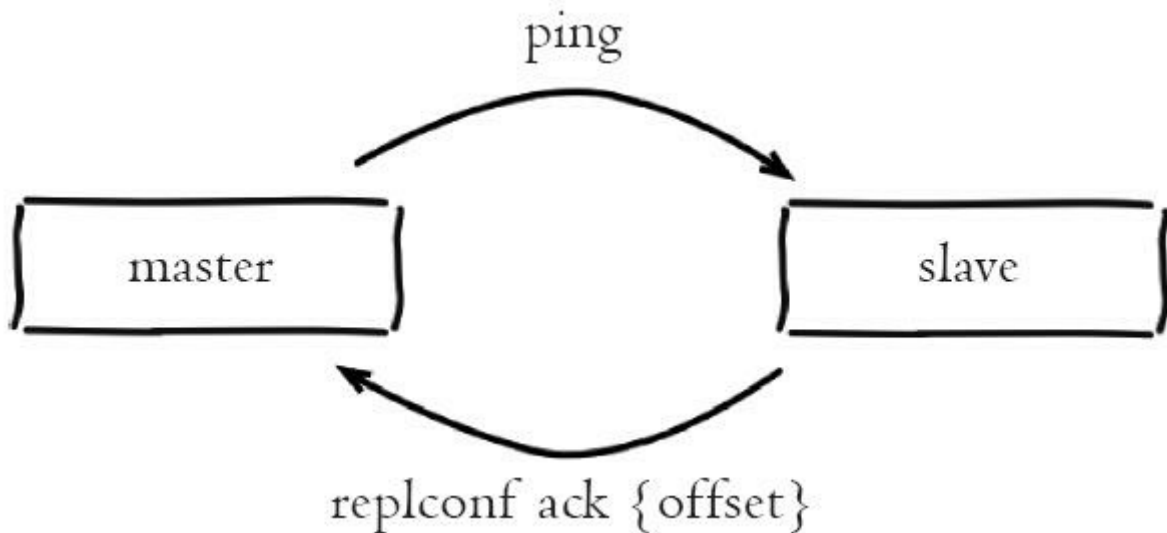
图6-17 主从心跳检测
