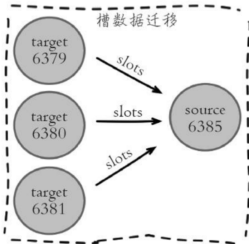
图10-22 槽和数据迁移到6385节点
