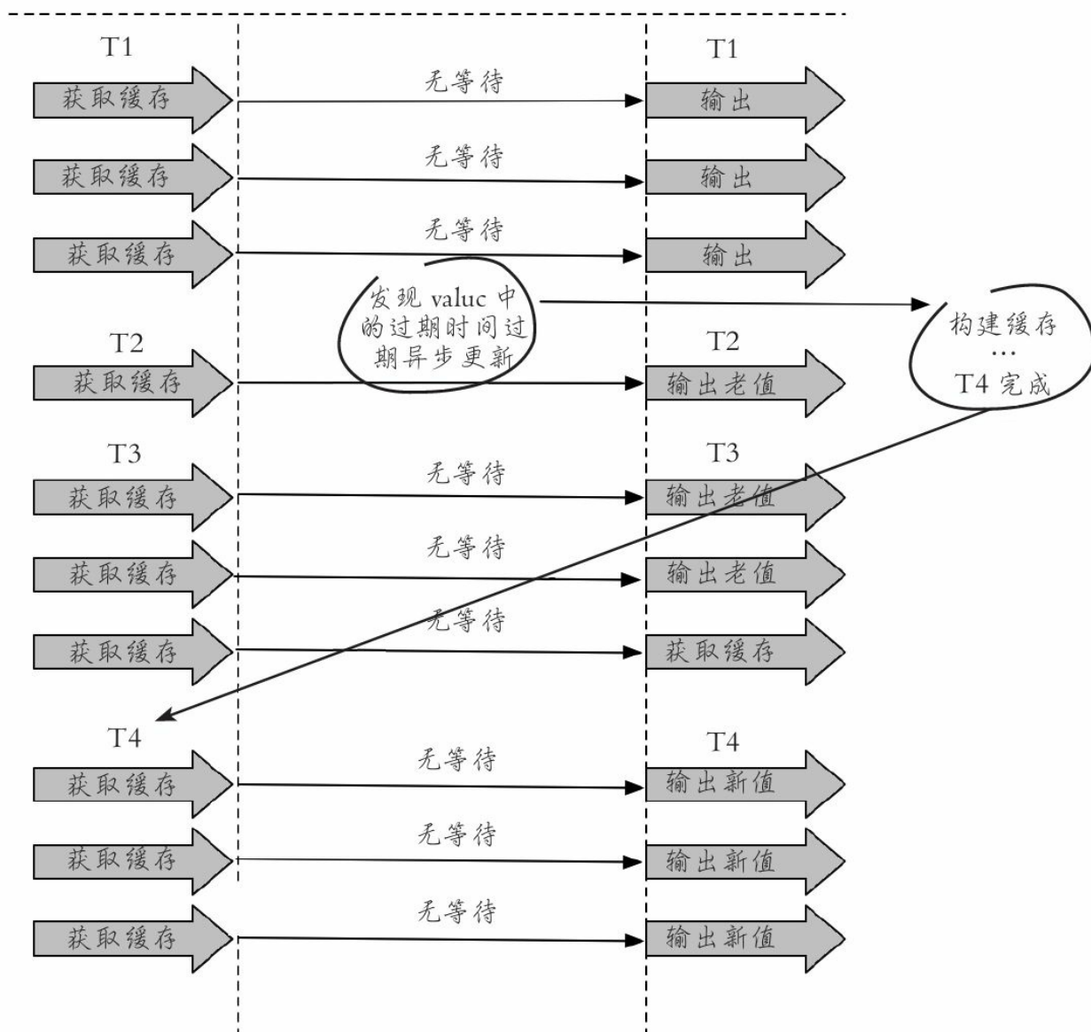
图11-18 “永远不过期”策略
