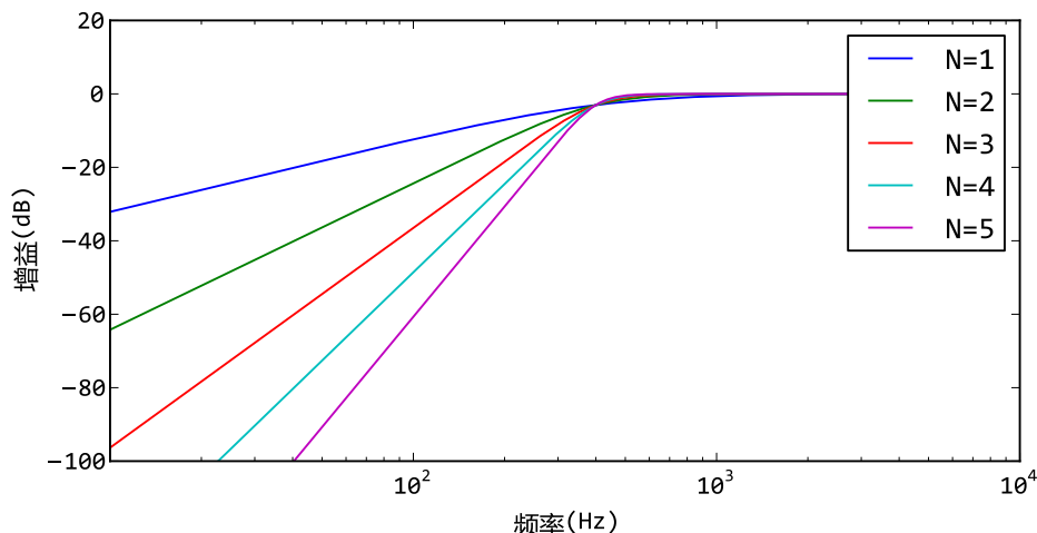
图 16.14 - iirfilter设计5个不同阶的IIR高通滤波器
