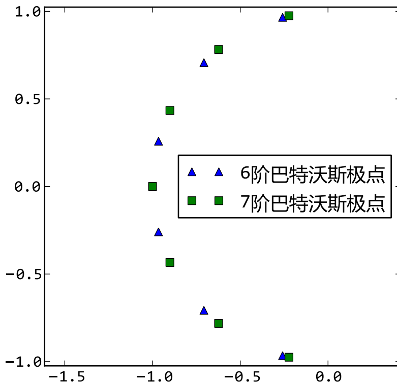
图 16.12 - 巴特沃斯低通滤波器在S复平面上的极点分布
