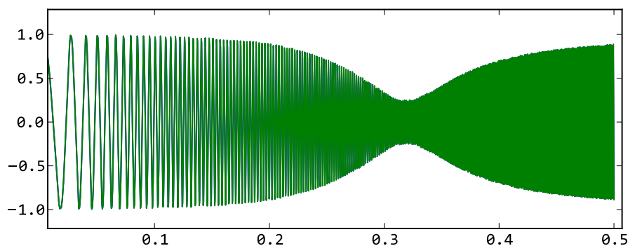
图 16.1 - 经过均衡滤波器之后的频率扫描波形
