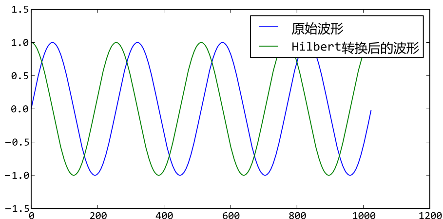
图 18.11 - Hilbert变换将正弦波变为余弦波
