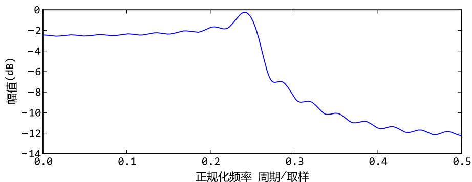
图 16.5 - 截取sinc函数正时间部分作为脉冲响应的低通滤波器
