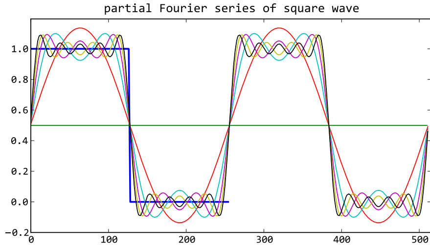
图 17.3 - 正弦波合成方波在跳变处出现都抖动
