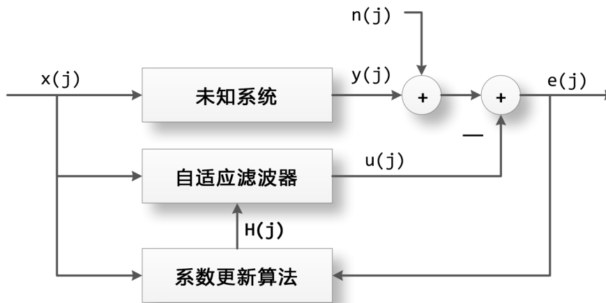
系统识别 (system identification)框图
