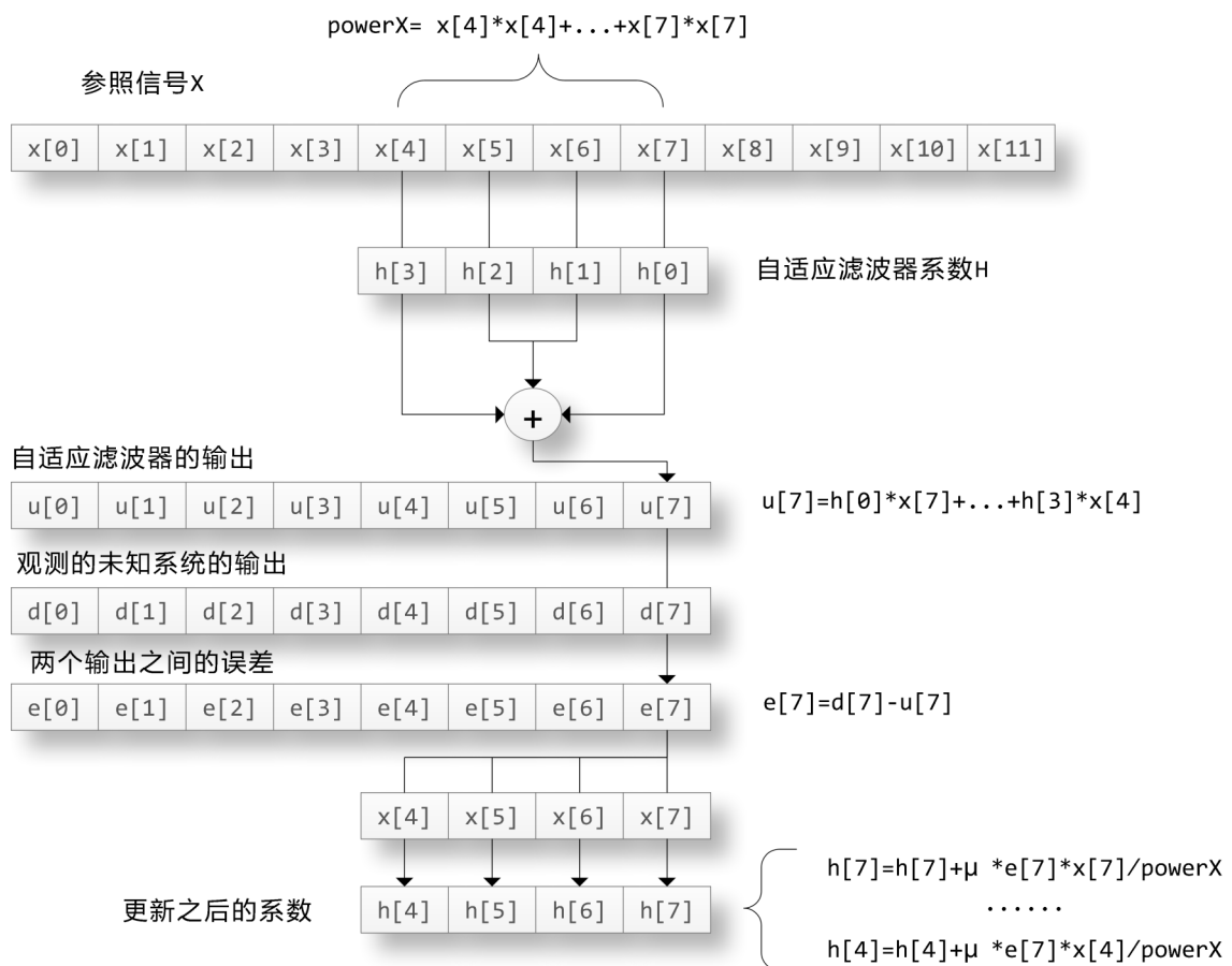
图 20.4 - NLMS算法示意图
