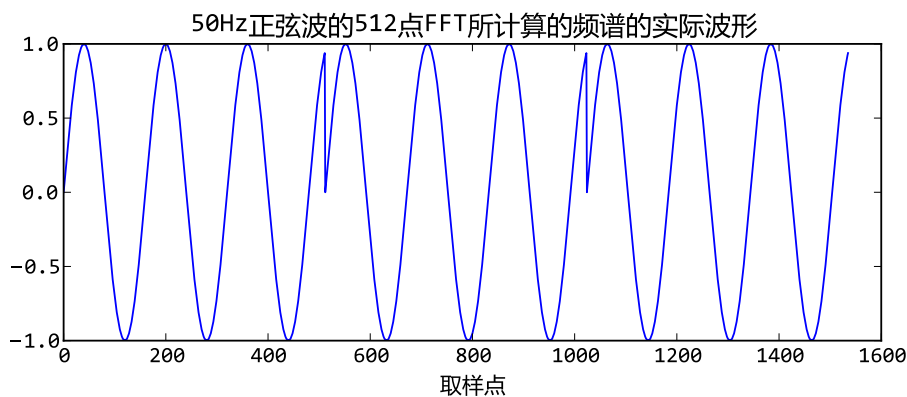
图 18.3 - 50Hz正弦波的512点FFT所计算的频谱的实际波形
