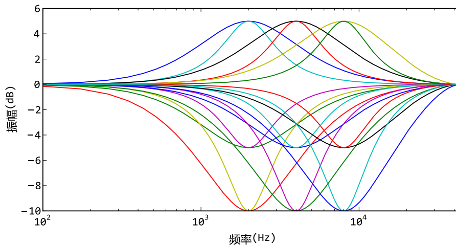
图 16.15 - 二次均衡滤波器的频率响应
