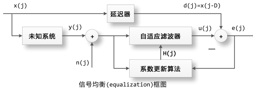
图 20.3 - 信号均衡(Equalization)框图
