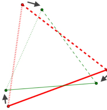
图 22.4 - 两个三角形决定一个2D仿射变换的六个参数
