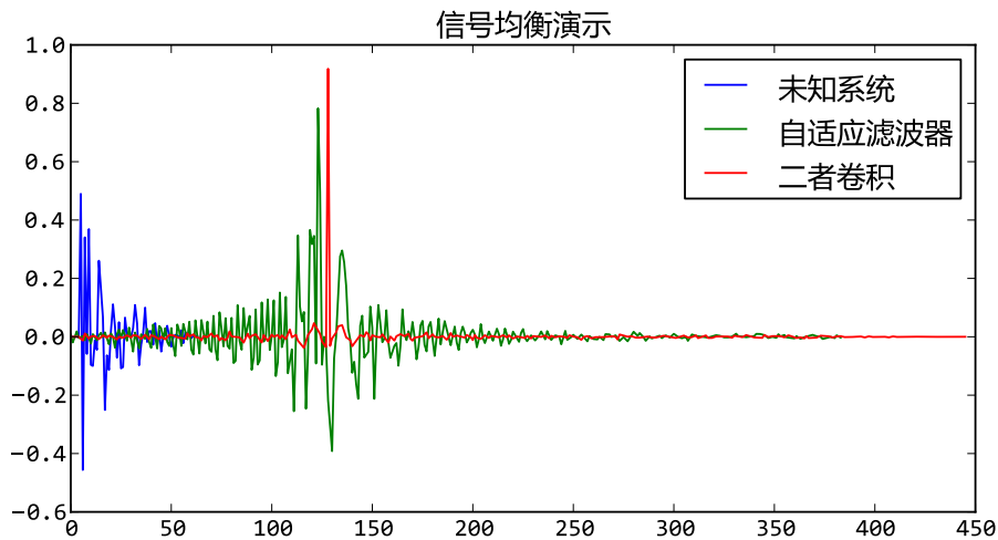
图 20.10 - 未知系统和自适应滤波器的级联(卷积)近似为标准延迟
