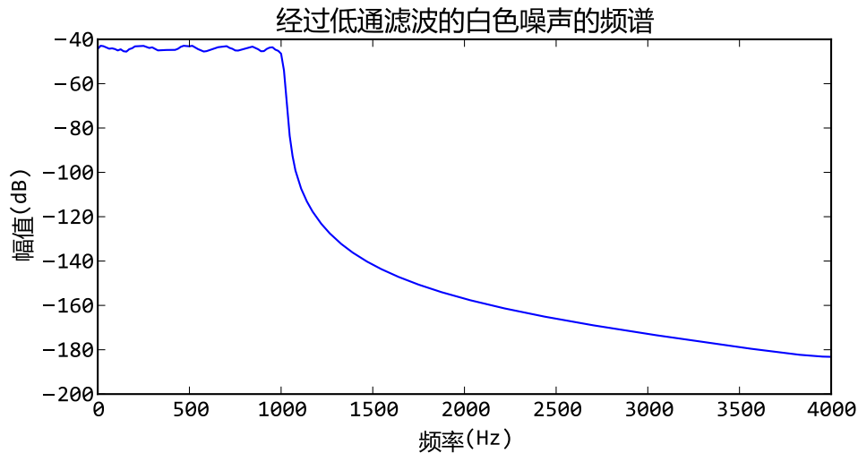
图 18.8 - 经过低通滤波器的白色噪声的频谱
