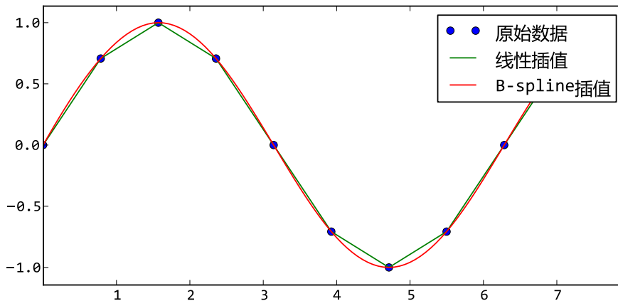
图 3.2 - 使用interpolate库对正弦波数据进行线性插值和B-Spline插值
