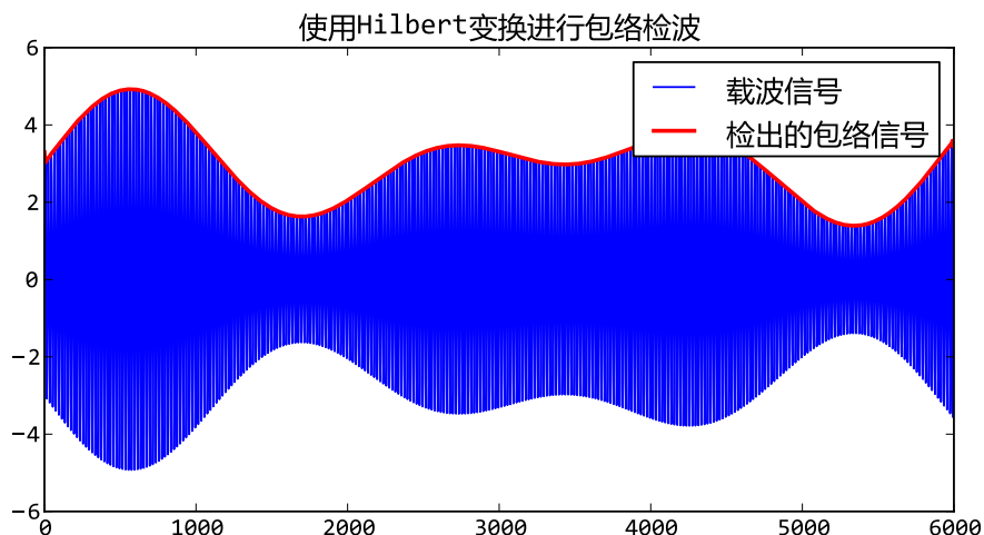
图 18.12 - 使用Hilbert变换对载波信号进行包络检波
