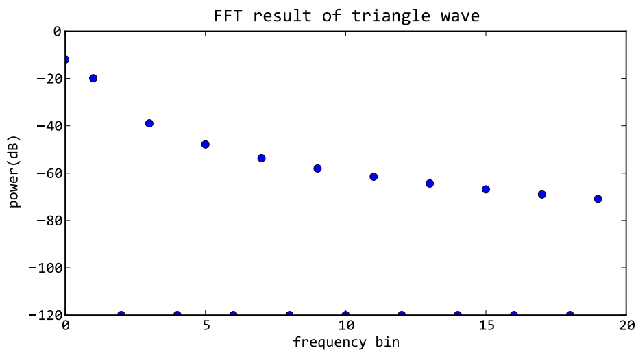
图 17.1 - 三角波的频谱
