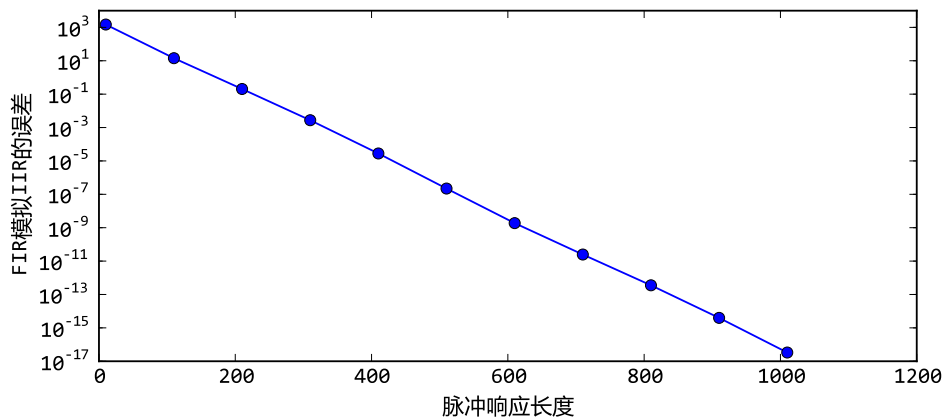
图 16.3 - 随着FIR滤波器的长度的增加误差呈指数减小
