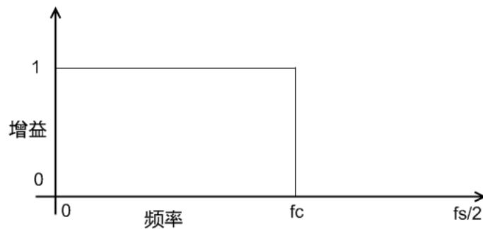
图 16.4 - 理想低通滤波器的频率响应
