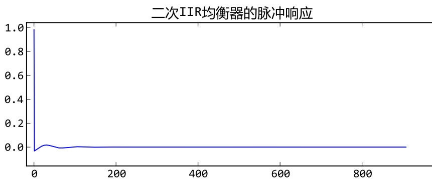
图 16.2 - 均衡滤波器的脉冲响应
