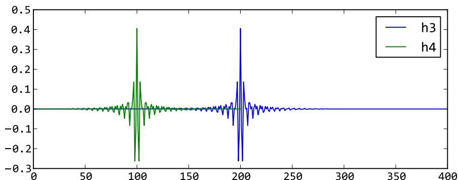
图 16.11 - 级联的滤波器和remez设计的带通滤波器的脉冲响应近似
