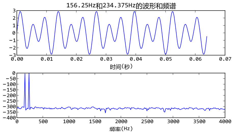
图 18.1 - 使用FFT计算正弦波的频谱
