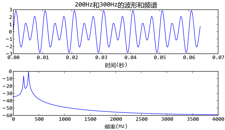
图 18.2 - 非完整周期的正弦波经过FFT变换之后出现频谱泄漏
