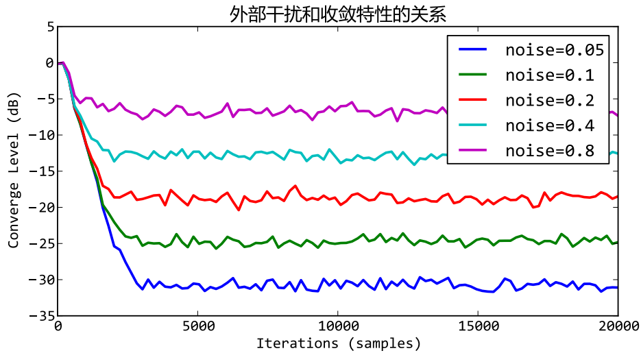
图 20.8 - 外部干扰噪声和收敛速度的关系
