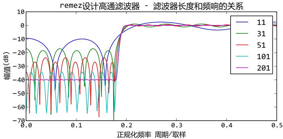
图 16.8 - remez设计的高通滤波器，长度越长频率响应越接近设计值
