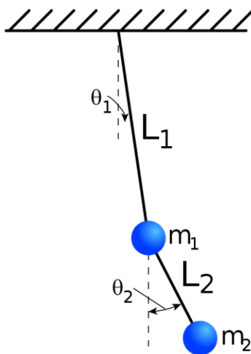
图 21.4 - 双摆装置示意图
