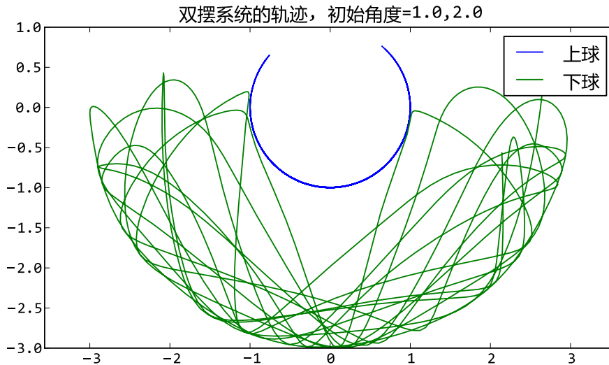
图 21.6 - 大初始角度时双摆的摆动轨迹呈现混沌现象
