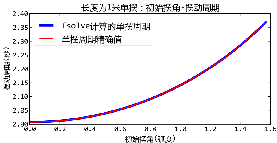
图 21.3 - 单摆的摆动周期和初始角度的关系
