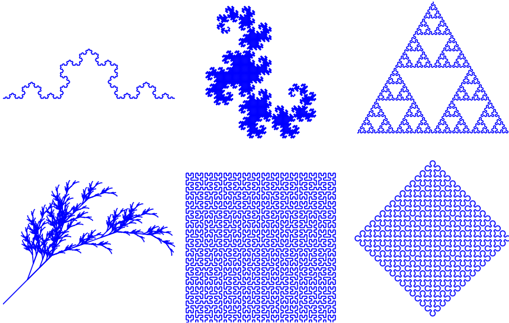
图 22.8 - 几种L-System的迭代图案
