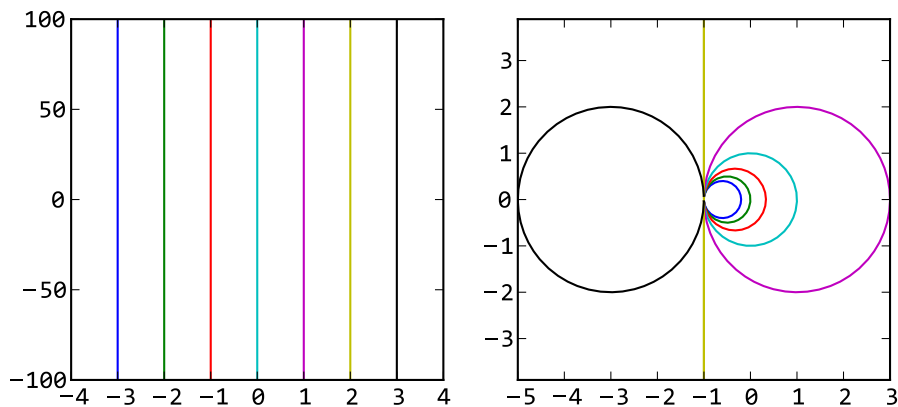
图 16.13 - 双线性变换将s平面(左图)上的竖线变换为z平面上的圆(右图)
