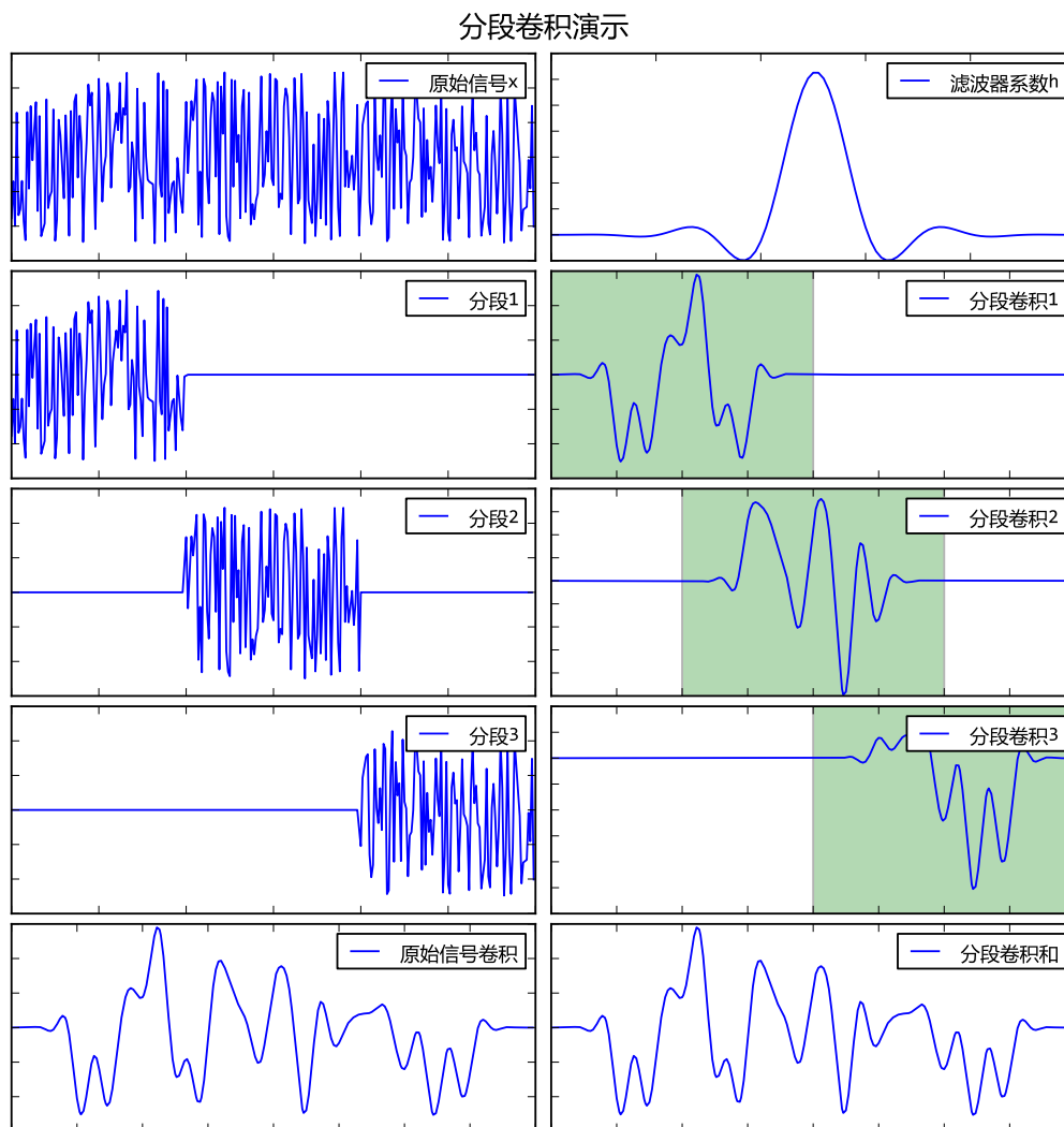
图 18.10 - 分段卷积的过程演示
