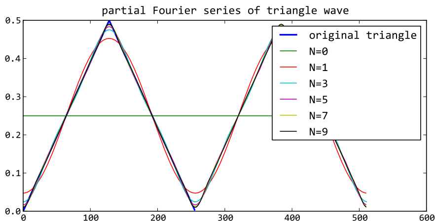
图 17.2 - 部分频谱重建的三角波
