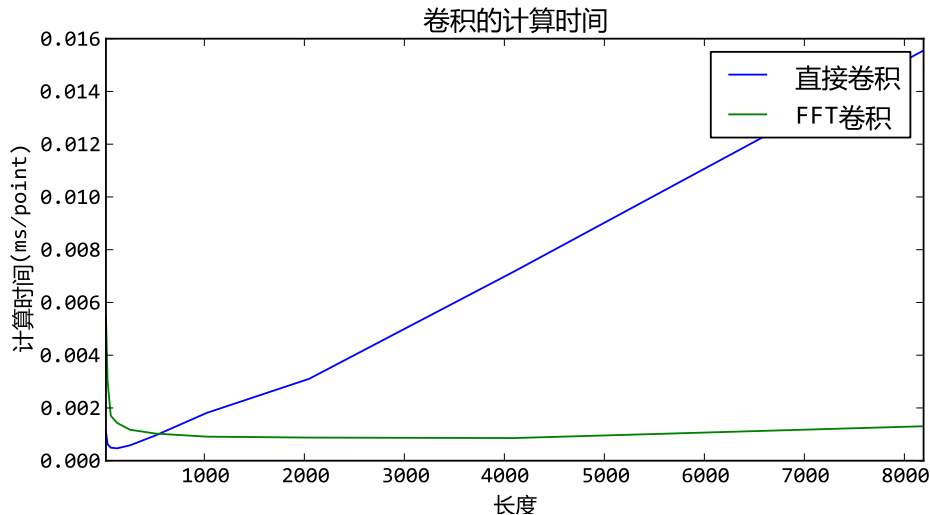
图 18.9 - 用FFT计算卷积和直接卷积的时间复杂度比较
