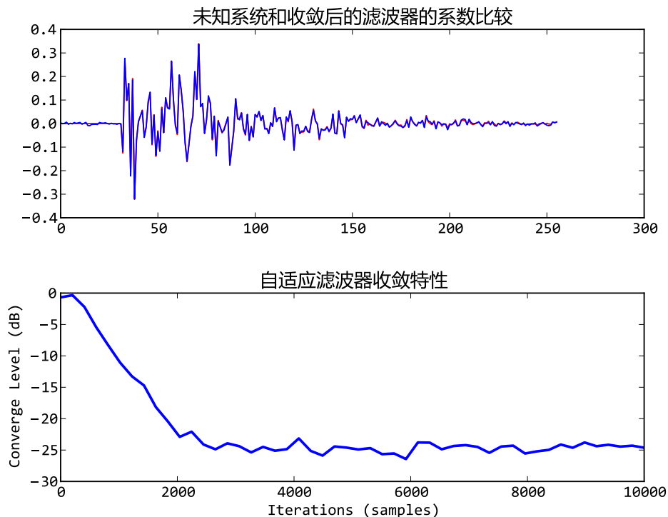
图 20.6 - 自适应滤波器收敛之后的系数和收敛速度
