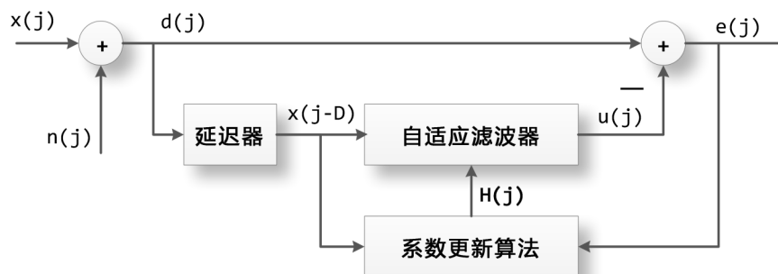
信号预测 (prediction)框图
