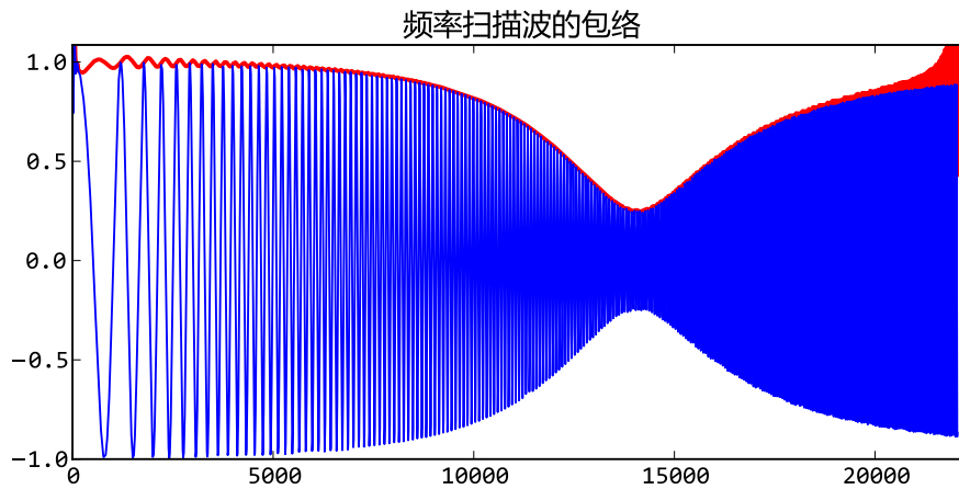
图 18.13 - 使用Hilbert变换对频率扫描波进行包络检波
