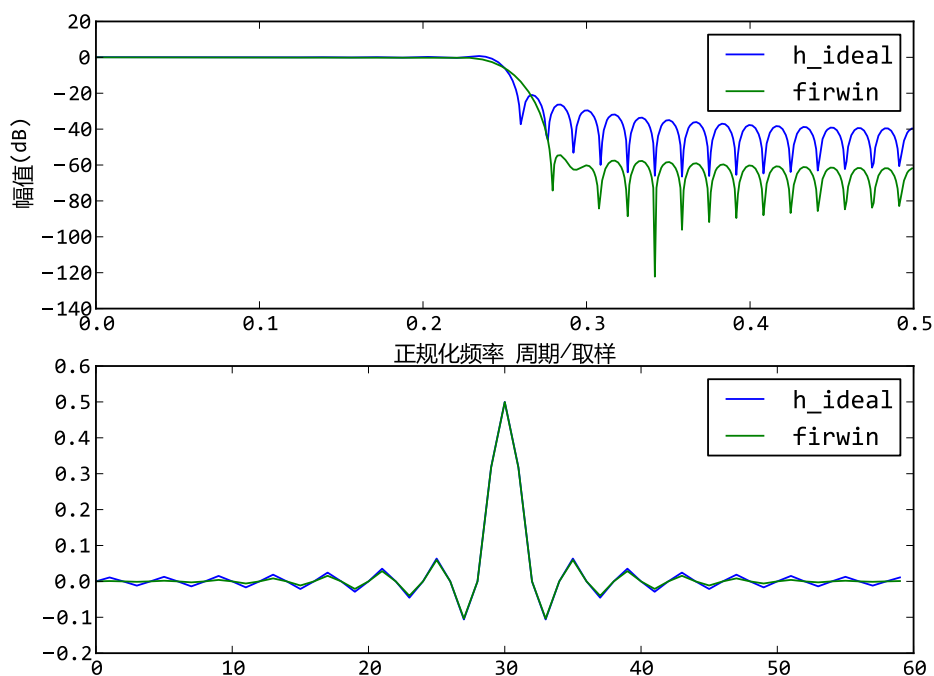
图 16.7 - firwin使用窗函数设计的低通滤波器的频率响应和脉冲响应
