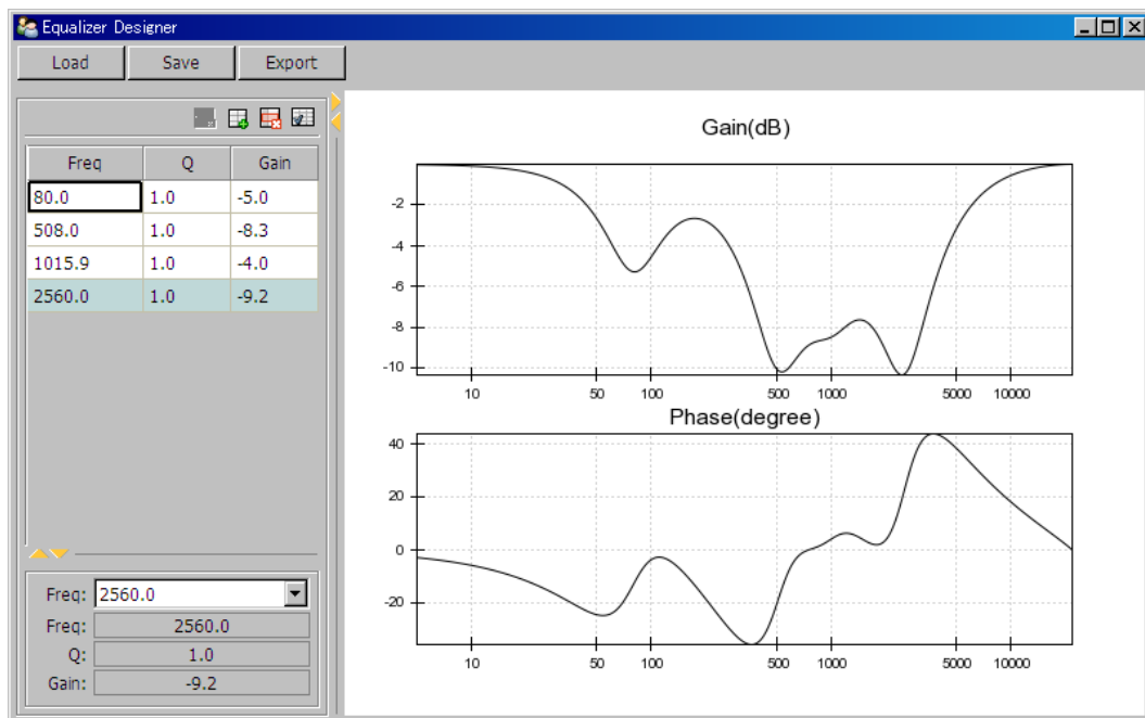
图 16.16 - 二次均衡器设计工具的界面
