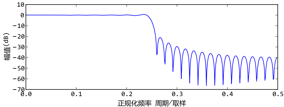
图 16.6 - 对称截取sinc函数的低通滤波器
