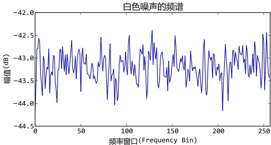
图 18.7 - 白色噪声的频谱接近水平直线(注意Y轴的范围)
