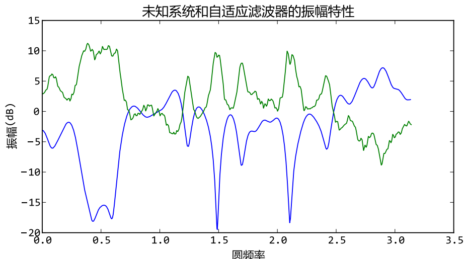
图 20.11 - 未知系统和自适应滤波器的频率响应正好相反
