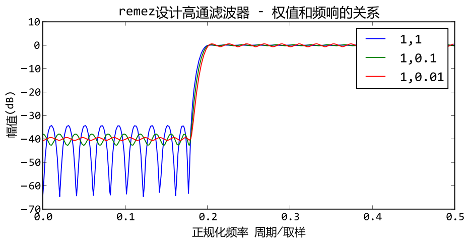
图 16.9 - remez设计滤波器时权值影响频率响应
