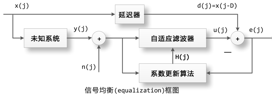
图 20.9 - 信号均衡(Equalization)框图
