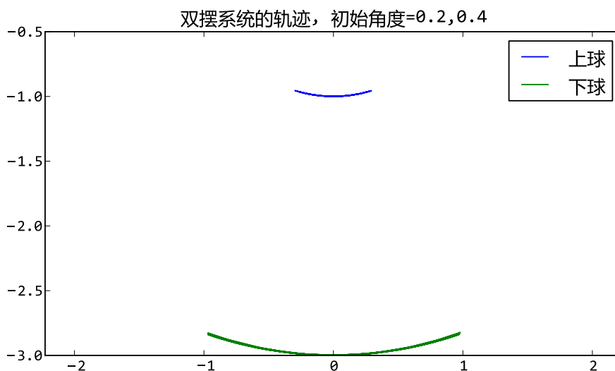
图 21.5 - 初始角度微小时的双摆的摆动轨迹
