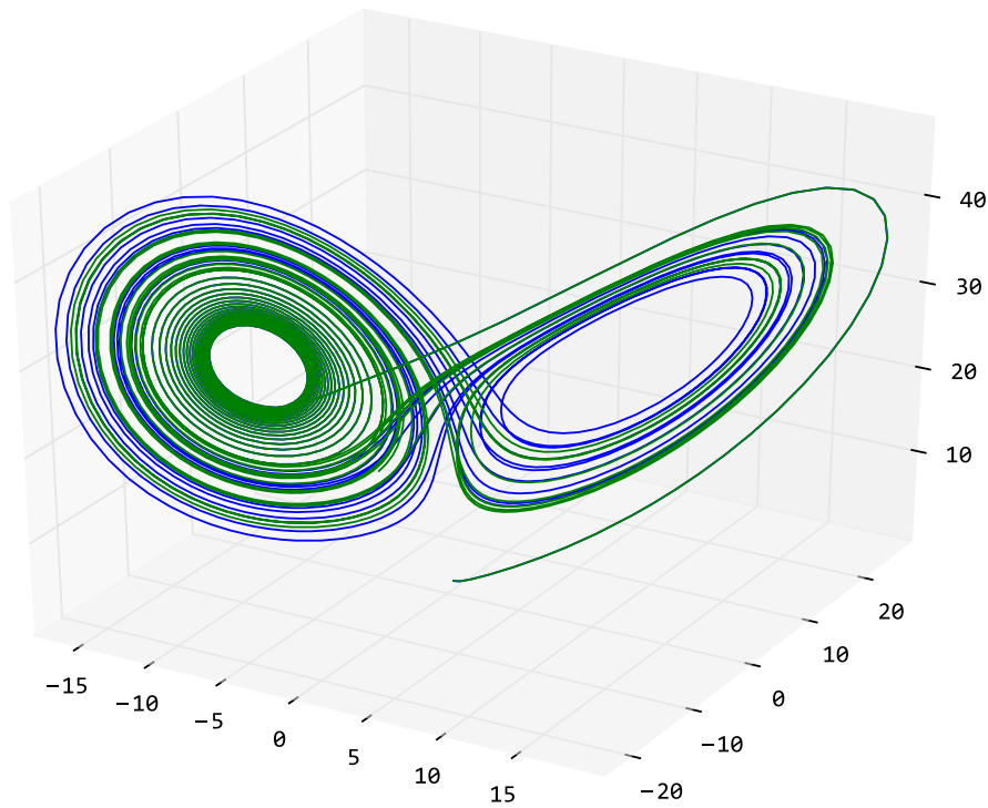
图 3.4 - 用odeint函数对洛伦兹吸引子微分方程进行数值求解所得到的运动轨迹
