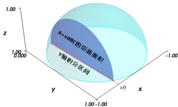
图 3.3 - 半球体积的双重定积分示意图
