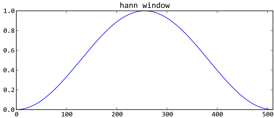
图 18.4 - hann窗函数
