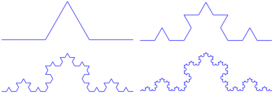
图 22.7 - 使用F+F--F+F迭代的分形图案
