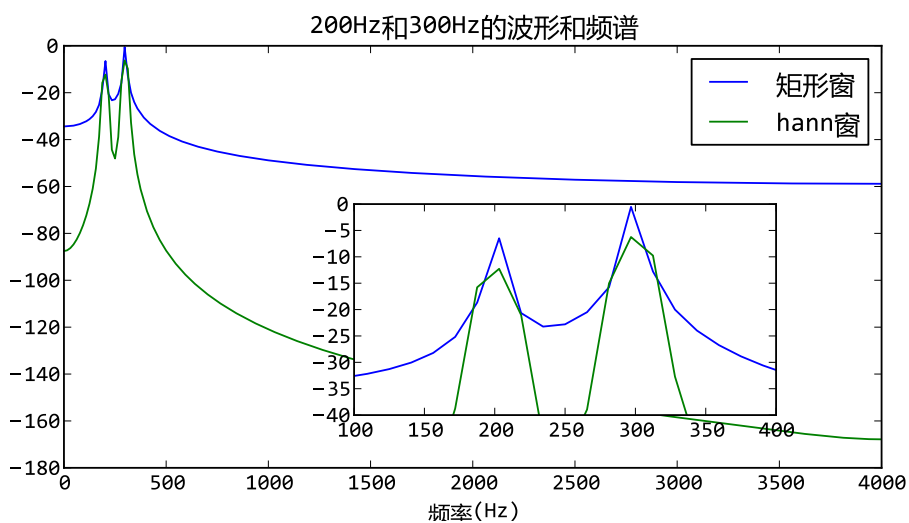
图 18.6 - 加hann窗前后的频谱，hann窗能降低频谱泄漏
