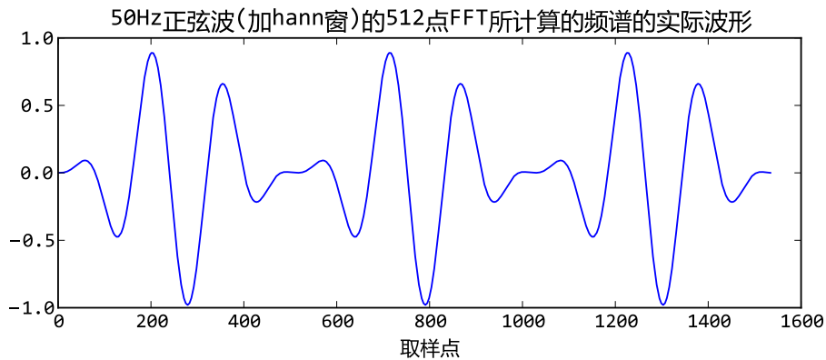
图 18.5 - 加hann窗的50Hz正弦波的512点FFT所计算的实际波形
