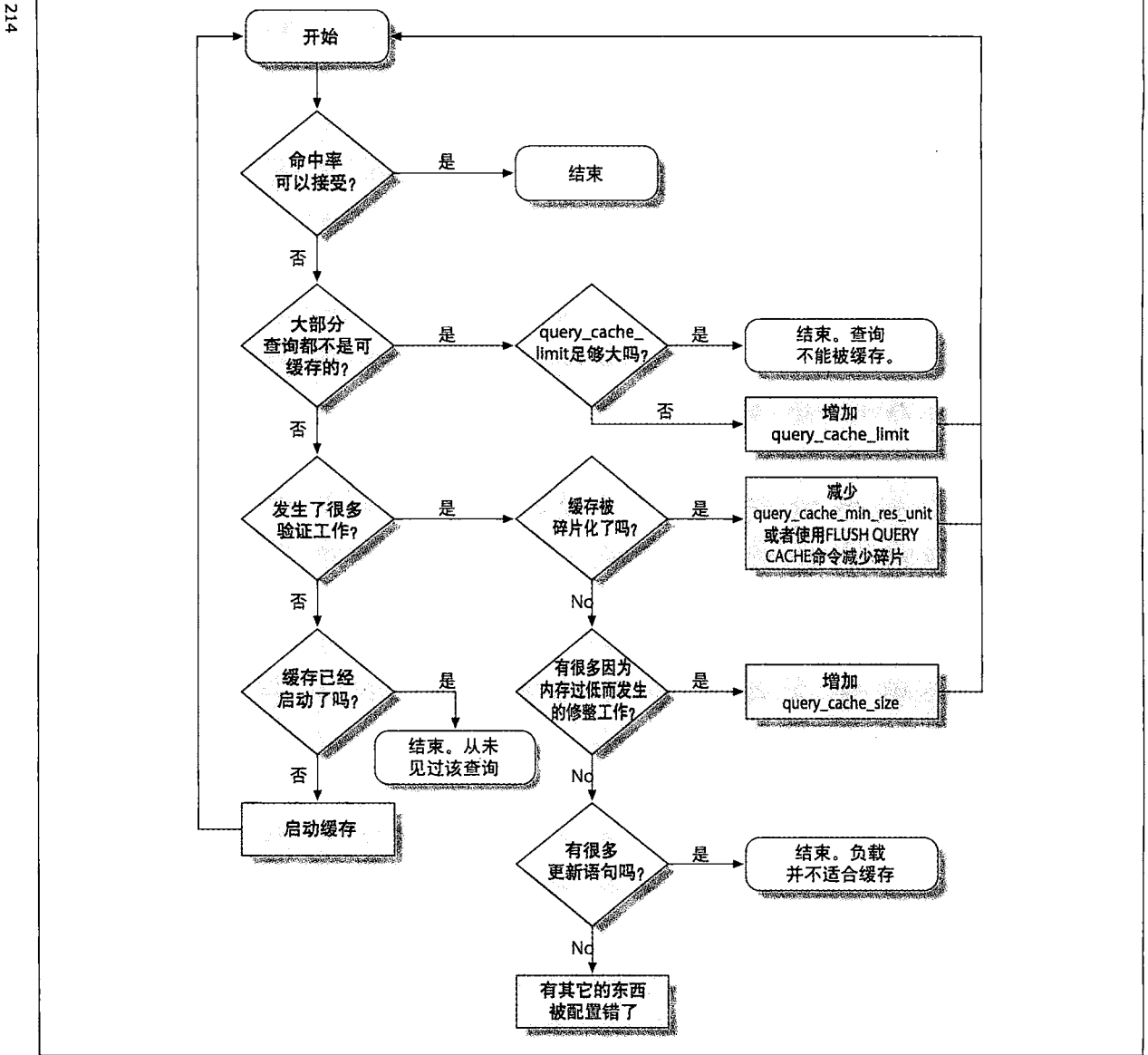
图 5-3：如何分析调整查询缓存
