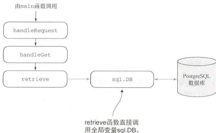
图 8-3 简单 Web 服务在处理 GET 请求时的函数调用流程图
