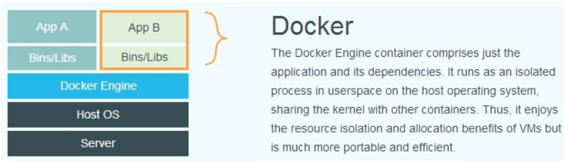
图 1.4.1.2 - Docker
