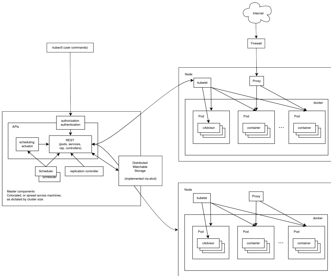
图 1.21.5.1 - Kubernetes 架构
