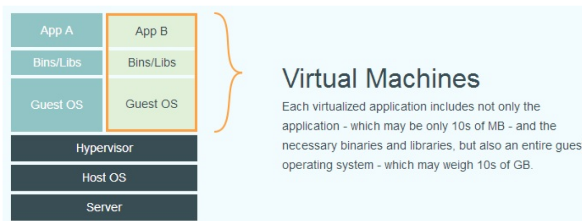
图 1.4.1.1 - 传统虚拟化
