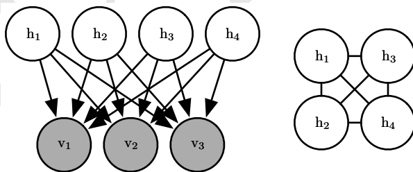
图 19.2: 包含四个隐藏单元的二值稀疏编码的图结构。(左) p(\mathbf{h}, \mathbf{v}) 的图结构。要注意边是有向的, 每两个隐藏单元都是每个可见单元的共父。(右) p(\mathbf{h} | \mathbf{v}) 的图结构。为了解释共父之间的活跃路径, 后验分布所有隐藏单元之间都有边。
