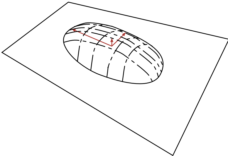
图 13.3: 平坦的高斯能够描述一个低维流形附近的概率密度。此图表示了“流形平面”上“馅饼”的上半部分, 并且这个平面穿过了馅饼的中心。正交于流形方向(指向平面外的箭头方向)的方差非常小, 可以被视为是“噪声”, 其他方向(平面内的箭头)的方差则很大, 对应了“信号”以及降维数据的坐标系统。
