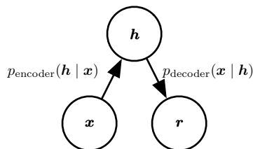
图 14.2: 随机自编码器的结构, 其中编码器和解码器包括一些噪声注入, 而不是简单的函数。这意味着可以将它们的输出视为来自分布的采样 (对于编码器是 p_{\text{encoder}}(\mathbf{h} | \mathbf{x}) , 对于解码器是 p_{\text{decoder}}(\mathbf{x} | \mathbf{h}) )。
