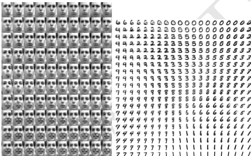
图 20.6: 由变分自编码器学习的高维流形在 2 维坐标系中的示例 (Kingma and Welling, 2014a)。我们可以在纸上直接绘制两个可视化的维度，因此可以使用 2 维潜在编码训练模型来了解模型的工作原理（即使我们认为数据流形的固有维度要高得多）。图中所示的图像不是来自训练集的样本，而是仅仅通过改变 2 维“编码” z ，由模型 p(\mathbf{x} | z) 实际生成的图像 \mathbf{x} （每个图像对应于“编码” z 位于 2 维均匀网格的不同选择）。(左) Frey 人脸流形的 2 维映射。其中一个维度（水平）已发现大致对应于面部的旋转，而另一个（垂直）对应于情绪表达。(右) MNIST 流形的 2 维映射。
