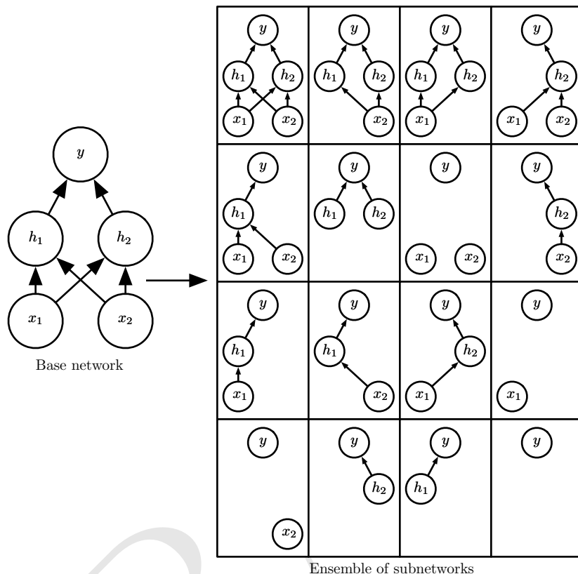
图 7.6: Dropout 训练由所有子网络组成的集成，其中子网络通过从基本网络中删除非输出单元构建。我们从具有两个可见单元和两个隐藏单元的基本网络开始。这四个单元有十六个可能的子集。右图展示了从原始网络中丢弃不同的单元子集而形成的所有十六个子网络。在这个小例子中，所得到的大部分网络没有输入单元或没有从输入连接到输出的路径。当层较宽时，丢弃所有从输入到输出的可能路径的概率变小，所以这个问题不太可能在出现层较宽的网络中。
