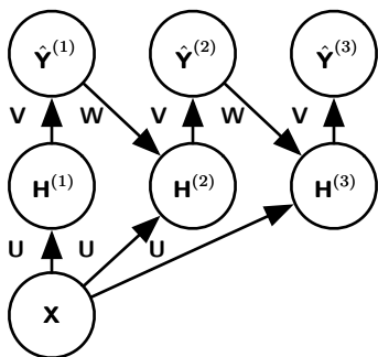
图 9.17: 用于像素标记的循环卷积网络的示例。输入是图像张量 \mathbf{X} ，它的轴对应图像的行、列和通道（红，绿，蓝）。目标是输出标签张量 \hat{\mathbf{Y}} ，它遵循每个像素的标签的概率分布。该张量的轴对应图像的行、列和不同类别。循环网络通过使用 \hat{\mathbf{Y}} 的先前的估计作为创建新估计的输入，来迭代地改善其估计，而不是单次输出 \hat{\mathbf{Y}} 。每个更新的估计使用相同的参数，并且估计可以如我们所愿地被改善任意多次。每一步使用的卷积核张量 \mathbf{U} ，是用来计算给定输入图像的隐藏表示的。核张量 \mathbf{V} 用于产生给定隐藏值时标签的估计。除了第一步之外，核 \mathbf{W} 都对 \hat{\mathbf{Y}} 进行卷积来提供隐藏层的输入。在第一步中，此项由零代替。因为每一步使用相同的参数，所以这是一个循环网络的例子，如第十章所述。
