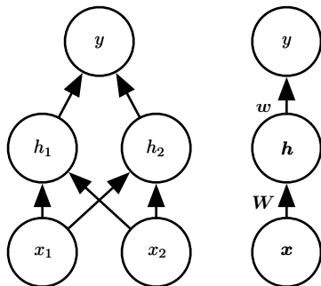
图 6.2: 使用两种不同样式绘制的前馈网络的示例。具体来说, 这是用来解决 XOR 问题的前馈网络。它有单个隐藏层, 包含两个单元。(左) 在这种样式中, 我们将每个单元绘制为图中的一个节点。这种风格是清楚而明确的, 但对于比这个例子更大的网络, 它可能会消耗太多的空间。(右) 在这种样式中, 我们将表示每一层激活的整个向量绘制为图中的一个节点。这种样式更加紧凑。有时, 我们对图中的边使用参数名进行注释, 这些参数是用来描述两层之间的关系。这里, 我们用矩阵 W 描述从 x 到 h 的映射, 用向量 w 描述从 h 到 y 的映射。当标记这种图时, 我们通常省略与每个层相关联的截距参数。
