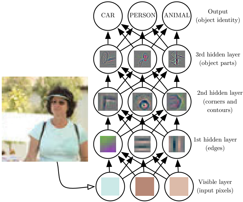
图 1.2: 深度学习模型的示意图。计算机难以理解原始感官输入数据的含义, 如表示为像素值集合的图像。将一组像素映射到对象标识的函数非常复杂。如果直接处理, 学习或评估此映射似乎是不可能的。深度学习将所需的复杂映射分解为一系列嵌套的简单映射 (每个由模型的不同层描述) 来解决这一难题。输入展示在 可见层 (visible layer), 这样命名的原因是因为它包含我们能观察到的变量。然后是一系列从图像中提取越来越多抽象特征的 隐藏层 (hidden layer)。因为它们的价值不在数据中给出, 所以将这些层称为“隐藏”; 模型必须确定哪些概念有利于解释观察数据中的关系。这里的图像是每个隐藏单元表示的特征的可视化。给定像素, 第一层可以轻易地通过比较相邻像素的亮度来识别边缘。有了第一隐藏层描述的边缘, 第二隐藏层可以容易地搜索可识别为角和扩展轮廓的边集合。给定第二隐藏层中关于角和轮廓的图像描述, 第三隐藏层可以找到轮廓和角的特定集合来检测特定对象的整个部分。最后, 根据图像描述中包含的对象部分, 可以识别图像中存在的对象。经 Zeiler and Fergus (2014) 许可转载此图。
