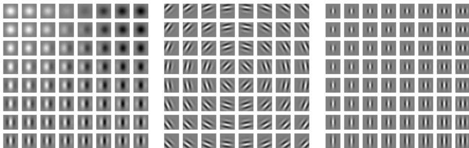
图 9.18: 具有各种参数设置的Gabor 函数。白色表示大的正权重, 黑色表示大的负权重, 背景灰色对应于零权重。(左) 控制坐标系的参数具有不同值的Gabor 函数, 这些参数包括: x_0 、 y_0 和 \gamma 。在该网格中的每个Gabor 函数被赋予和它在网格中的位置成比例的 x_0 和 y_0 的值, 并且 \tau 被选择为使得每个 Gabor 过滤器对从网格中心辐射出的方向非常敏感。对于其他两幅图, x_0 、 y_0 和 \gamma 固定为零。(中) 具有不同高斯比例参数 \beta_x 和 \beta_y 的Gabor 函数。当我们从左到右通过网格时, Gabor 函数被设置为增加宽度 (减少 \beta_x ); 当我们从上到下通过网格时, Gabor 函数被设置为增加高度 (减少 \beta_y )。对于其他两幅图, \beta 值固定为图像宽度的 1.5 倍。(右) 具有不同的正弦参数 f 和 \phi 的Gabor 函数。当我们从上到下移动时, f 增加; 当我们从左到右移动时, \phi 增加。对于其他两幅图, \phi 固定为 0, f 固定为图像宽度的 5 倍。
