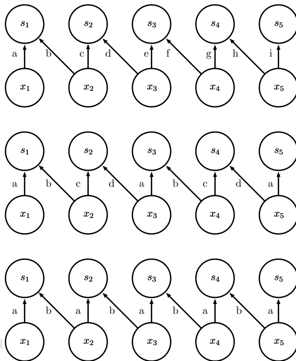
图 9.16: 局部连接层、平铺卷积和标准卷积的比较。当使用相同大小的核时,这三种方法在单元之间具有相同的连接。此图是对使用两个像素宽的核的说明。这三种方法之间的区别在于它们如何共享参数。(上)局部连接层根本没有共享参数。我们对每个连接使用唯一的字母标记,来表明每个连接都有它自身的权重。(中)平铺卷积有 t 个不同的核。这里我们说明 t=2 的情况。其中一个核具有标记为“a”和“b”的边,而另一个具有标记为“c”和“d”的边。每当我们在输出中右移一个像素后,我们使用一个不同的核。这意味着,与局部连接层类似,输出中的相邻单元具有不同的参数。与局部连接层不同的是,在我们遍历所有可用的 t 个核之后,我们循环回到了第一个核。如果两个输出单元间隔 t 个步长的倍数,则它们共享参数。(下)传统卷积等效于 t=1 的平铺卷积。它只有一个核,并且被应用到各个地方,我们在图中表示为在各处使用具有标记为“a”和“b”的边的核。
